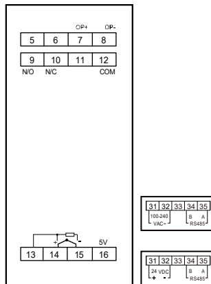
D71接线图
