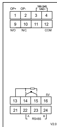
E71接线图
